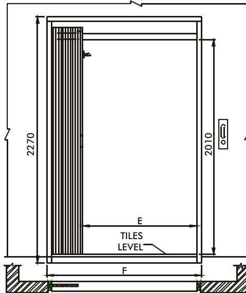
COLLAPSIBLE DOOR LANDING
